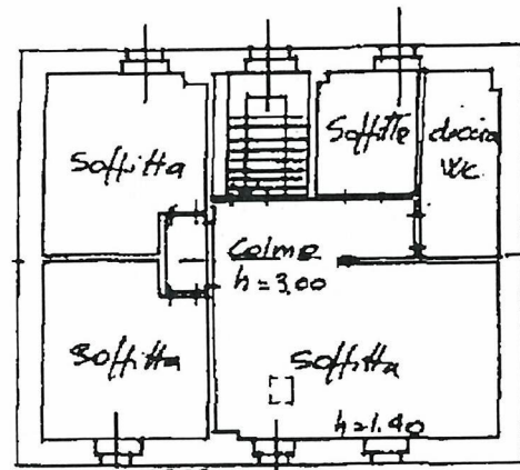
PIANO SOTTOTETTO
