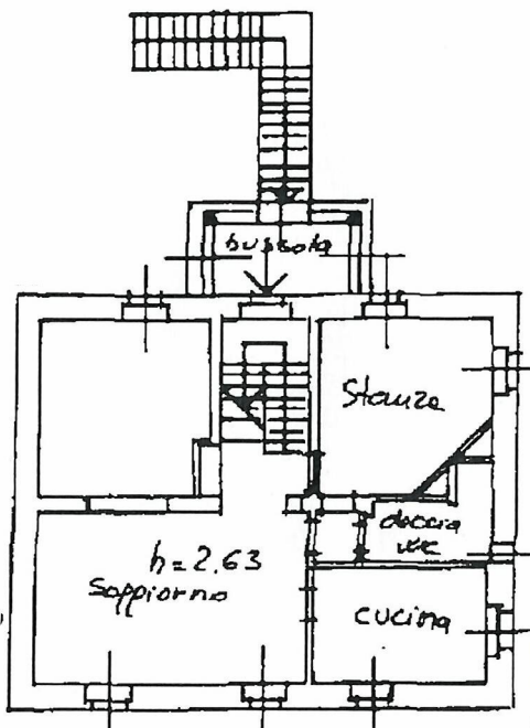
PIANO PRIMO
