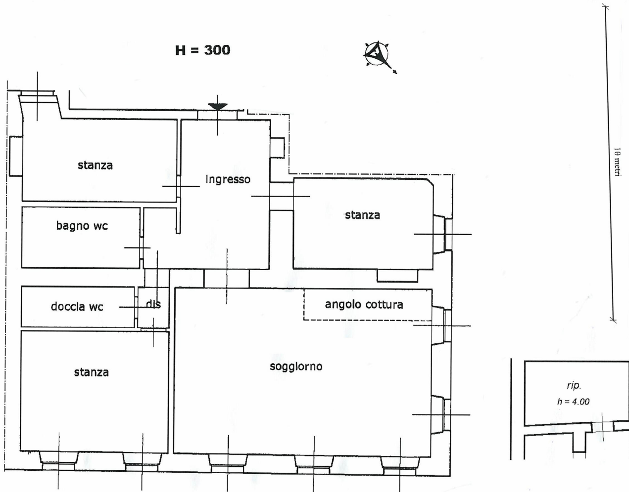
PIANTA PIANOTERRA
